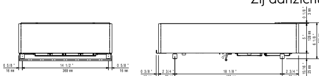
Zij aanzicht
